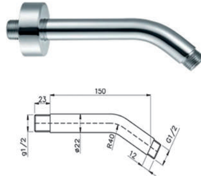
CR - AR - 15 - 206
