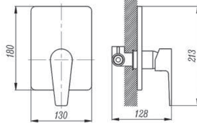
7465-321
