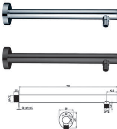
CR - AR - 40 - 201
