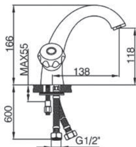
BR-101
