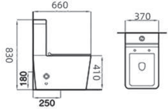
MODEL : A-8869
