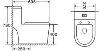
MODEL : 6264
