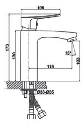
EUSH526-01
