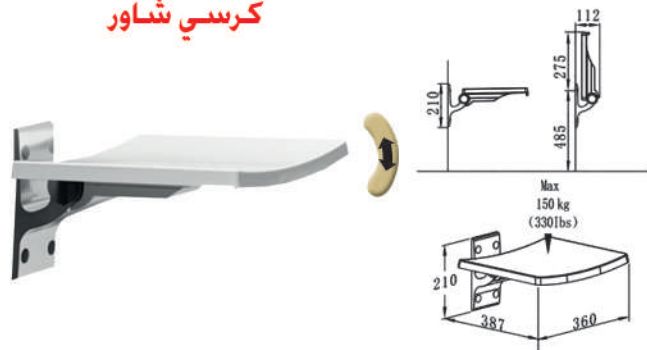
SA-A360
