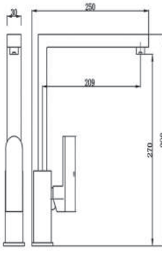
CR - 495 - 2
