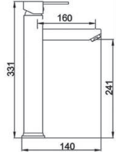
CR - 4801-H
