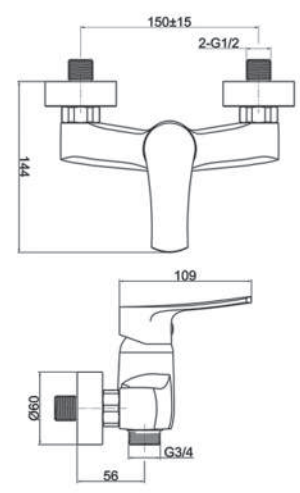
EUSH526-05
