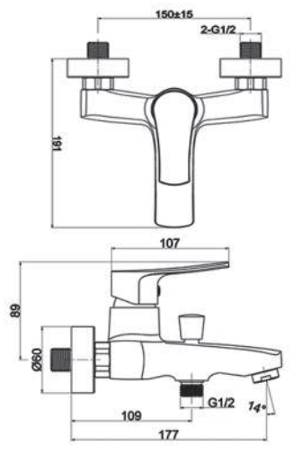
EUSH526-09
